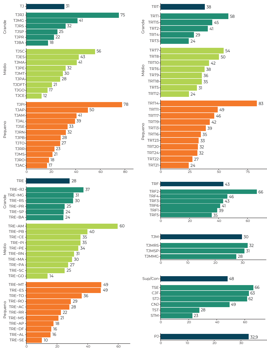
Figura 25: Consumo relativo de energia elétrica em quilowatts por área total em metros quadrados em 2023, por Tribunal/Conselho
