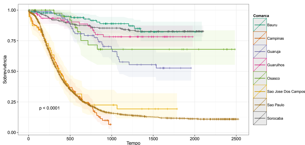
Figura 11.: Gráfico Kaplan-Meier do tempo dos processos de perda ou suspensão do poder familiar, da distribuição até a sentença, nas oito comarcas do estado de São Paulo com maior volume processual.
