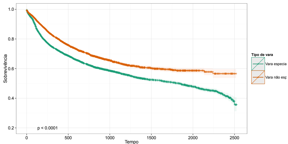
Figura 18.: Gráfico Kaplan-Meier do tempo dos processos de medidas protetivas à criança e adolescente, da distribuição até a sentença, comparando varas especializadas e não especializadas.
