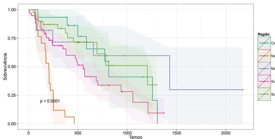
Figura 6.: Gráfico Kaplan-Meier do tempo dos processos de adoção, da distribuição até a sentença, por região, baseados nos dados das amostras. Cada curva está relacionada aos processos de uma determinada região, conforme a cor. Os traços verticais indicam os tempos de censura observados. As sombras que aparecem atrás das curvas são intervalos de confiança para as curvas a nível de confiança de 90%. O número próximo da letra "p" é o valor-p do teste que verifica se as curvas podem ser consideradas iguais. Quando esse número é pequeno (por exemplo, menor que 5%), rejeitamos a hipótese de que as curvas são iguais.
