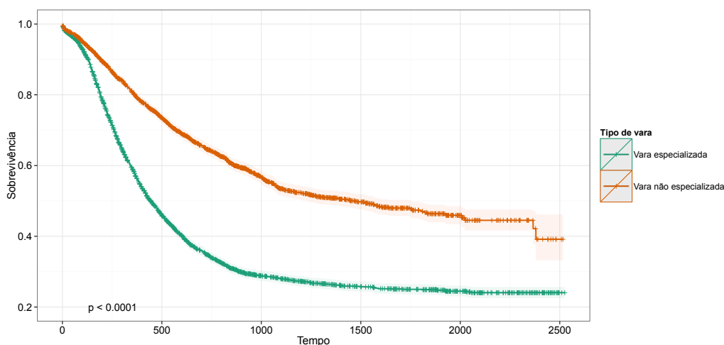
Figura 17.: Gráfico Kaplan-Meier do tempo dos processos de perda ou suspensão do poder familiar, da distribuição até a sentença, comparando varas especializadas e não especializadas.
