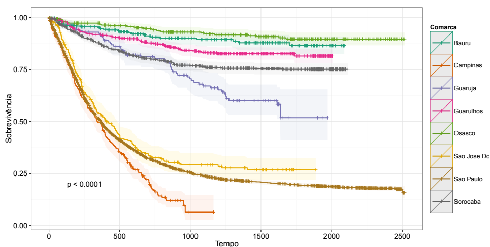
Figura 10.: Gráfico Kaplan-Meier do tempo dos processos de adoção ou adoção c/c destituição, da distribuição até a sentença, nas oito comarcas do estado de São Paulo com maior volume processual.
