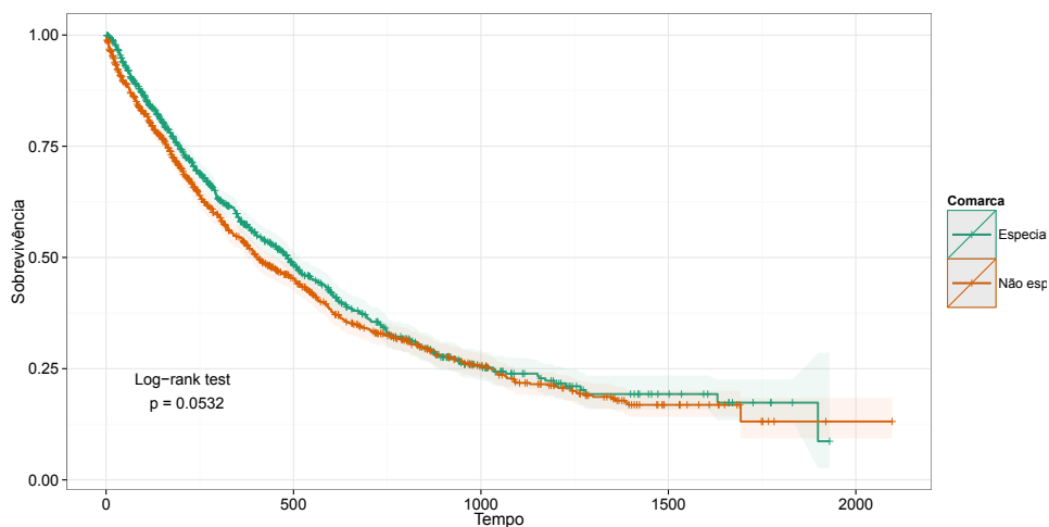
Figura 24.: Gráfico Kaplan-Meier do tempo dos processos de medidas protetivas à criança ou adolescente, da distribuição até a sentença, comparando varas especializadas e não especializadas.
