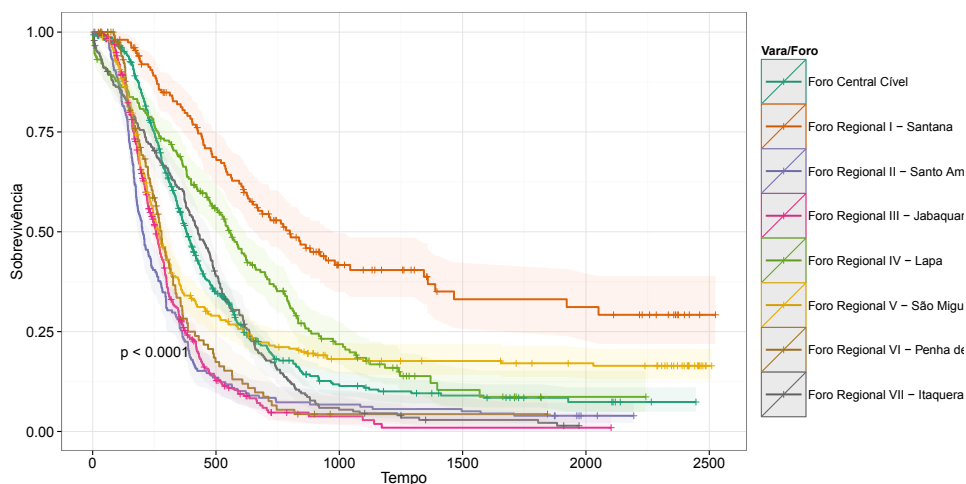
Figura 14.: Gráfico Kaplan-Meier do tempo dos processos de perda ou suspensão do poder familiar, da distribuição até a sentença, nas varas ou foros do município de São Paulo com maior volume processual.
