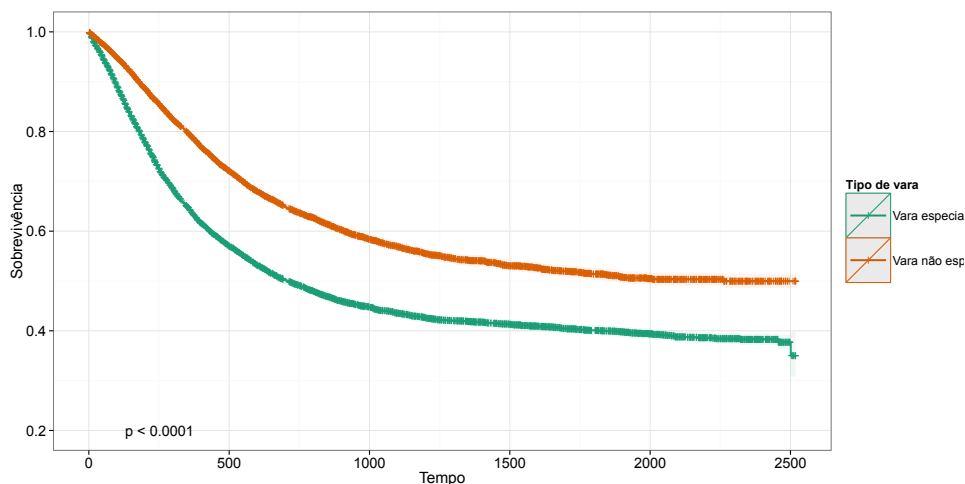
Figura 16.: Gráfico Kaplan-Meier do tempo dos processos de adoção ou adoção c/c destituição, da distribuição até a sentença, comparando varas especializadas e não especializadas.
