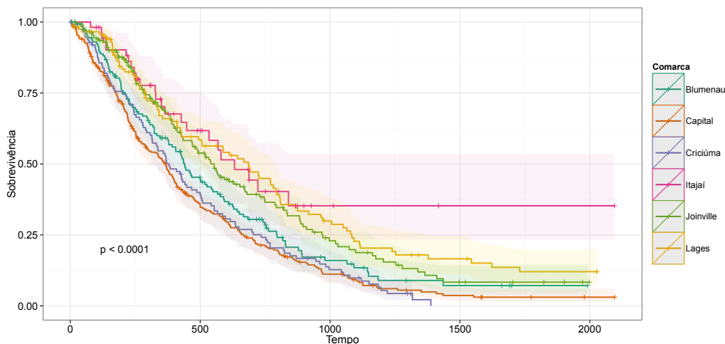
Figura 20.: Gráfico Kaplan-Meier do tempo dos processos de perda ou suspensão do poder familiar, da distribuição até a sentença, nas 6 comarcas do estado de Santa Catarina com maior volume processual.
