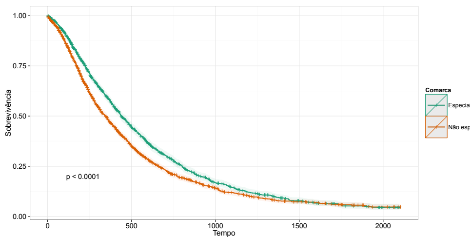
Figura 23.: Gráfico Kaplan-Meier do tempo dos processos de perda ou suspensão do poder familiar, da distribuição até a sentença, comparando varas especializadas e não especializadas.
