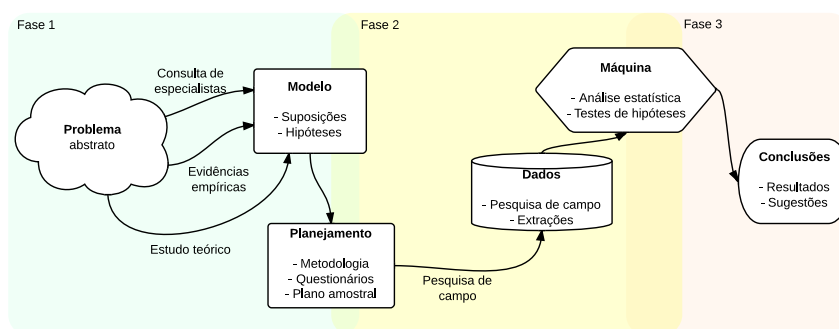
Figura 5.: Diagrama da metodologia empregada no projeto
