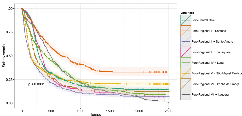
Figura 13.: Gráfico Kaplan-Meier do tempo dos processos de adoção ou adoção c/c destituição, da distribuição até a sentença, nas varas ou foros do município de São Paulo com maior volume processual.
