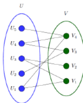
Figura 26.: Exemplo de grafo bipartido. No contexto do CNA, U representaria crianças e V pretendentes, e as arestas representariam os seus possíveis encontros.
