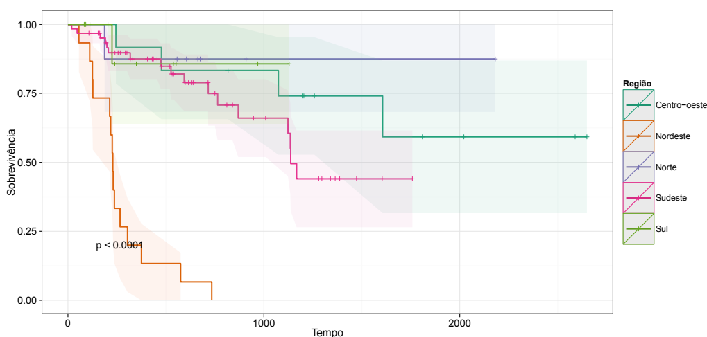
Figura 7.: Gráfico Kaplan-Meier do tempo dos processos de medidas protetivas ou destituição do poder familiar, da distribuição até a sentença, por região, baseados nos dados das amostras.
