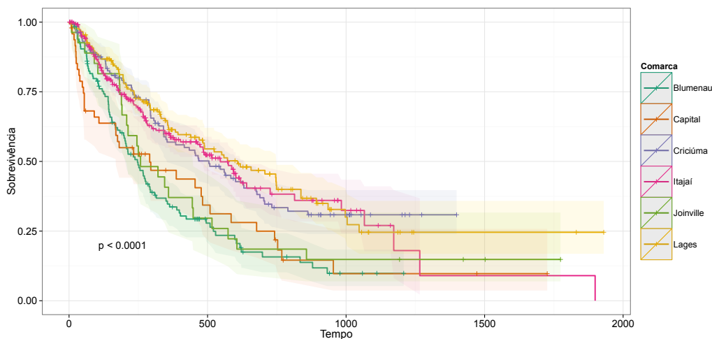
Figura 21.: Gráfico Kaplan-Meier do tempo dos processos de medidas protetivas à criança ou adolescente, da distribuição até a sentença, nas 6 comarcas do estado de Santa Catarina com maior volume processual.
