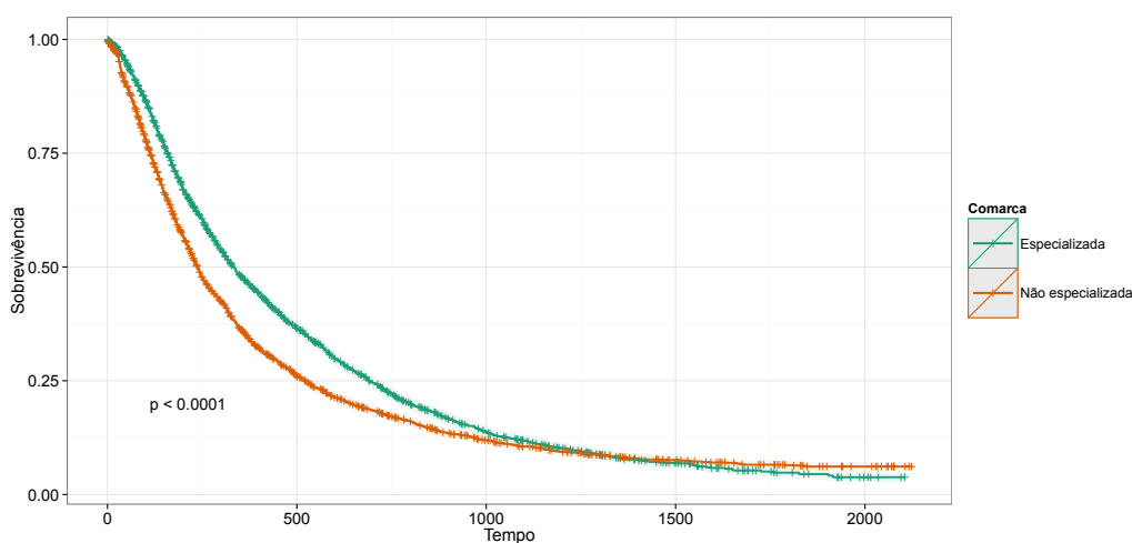
Figura 22.: Gráfico Kaplan-Meier do tempo dos processos de adoção ou adoção c/c destituição, da distribuição até a sentença, comparando varas especializadas e não especializadas.
