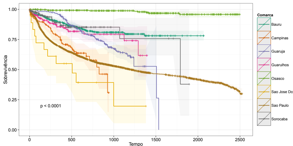
Figura 12.: Gráfico Kaplan-Meier do tempo dos processos de medidas protetivas à criança e adolescente, da distribuição até a sentença, nas oito comarcas do estado de São Paulo com maior volume processual.
