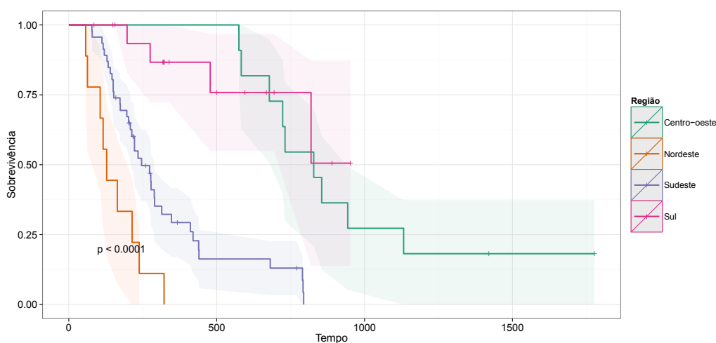
Figura 8.: Gráfico Kaplan-Meier do tempo dos processos de habilitação para adoção, da distribuição até a sentença, por região, baseados nos dados das amostras.
