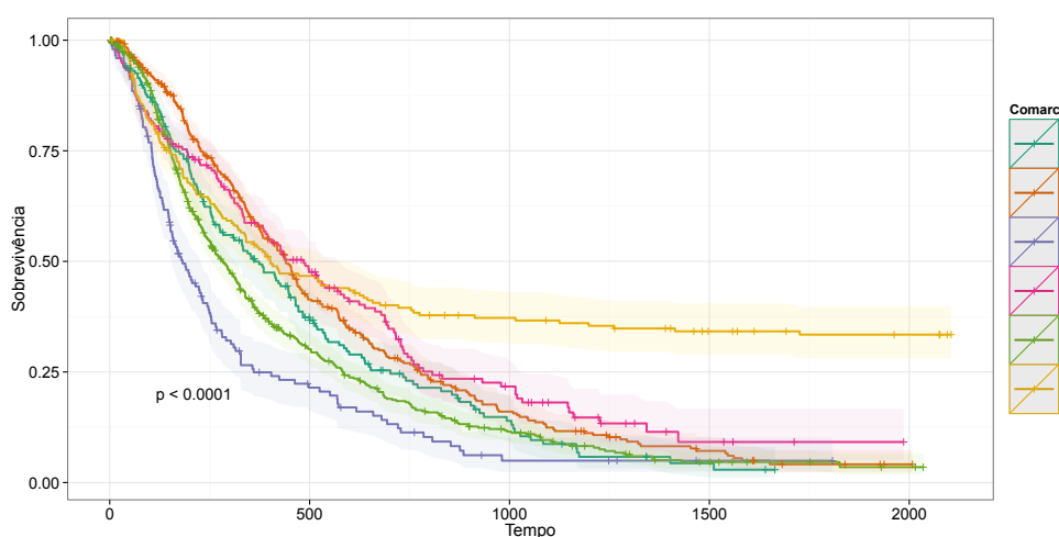
Figura 19.: Gráfico Kaplan-Meier do tempo dos processos de adoção ou adoção c/c destituição, da distribuição até a sentença, nas 6 comarcas do estado de Santa Catarina com maior volume processual.
