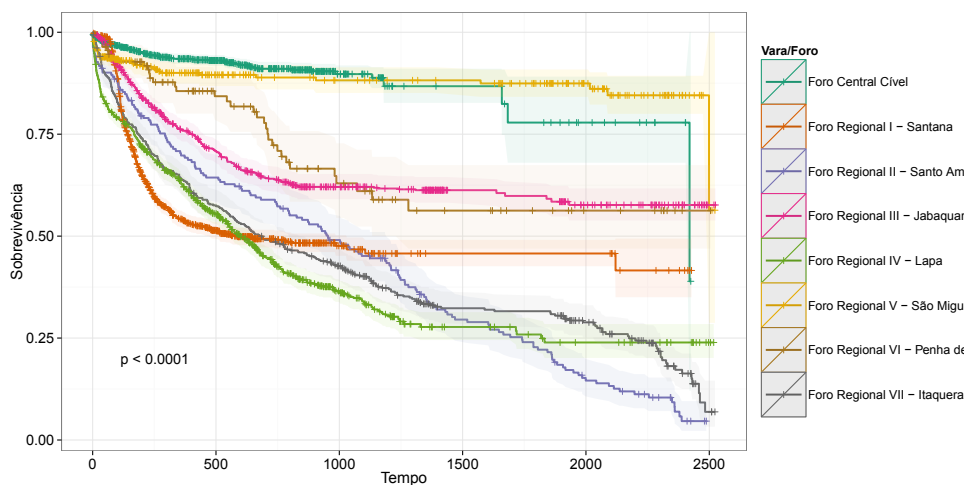
Figura 15.: Gráfico Kaplan-Meier do tempo dos processos de medidas protetivas à criança ou adolescente, da distribuição até a sentença, nas varas ou foros do município de São Paulo com maior volume processual.
